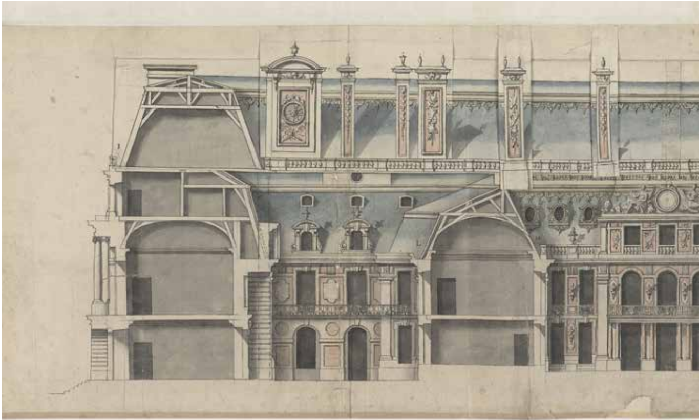
Projet de façade pour Versailles, du côté de la ville, avec surélévation des toits et cheminées » Archives nationales O1 1768, A1, n°2.
